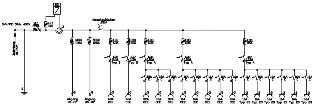
Stahlblechschrank
