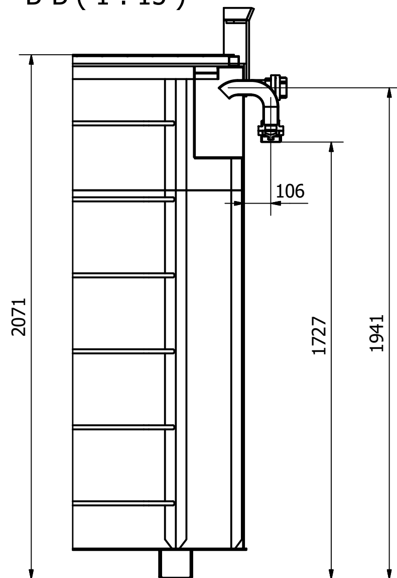
B-B ( 1 : 15 )
