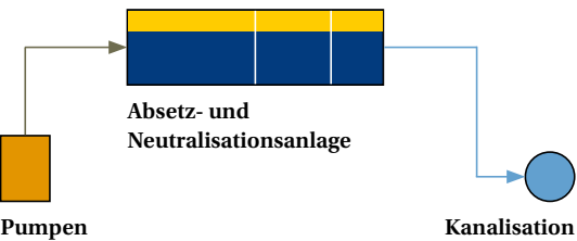
BEISPIEL 1 Kompaktlösung, bis 40 m³ in Kanalisation / 24 m³ ins Gewässer
