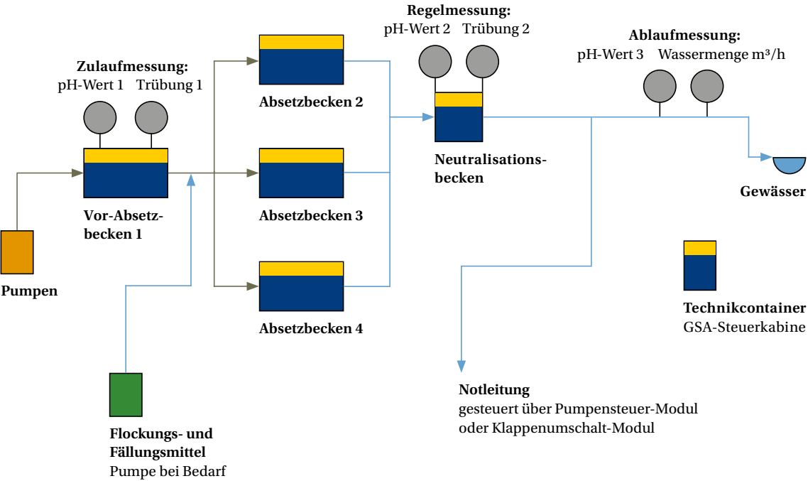
BEISPIEL 2 Mehrbeckenanlage, ab 40 m³ in Kanalisation / 24 m³ ins Gewässer
